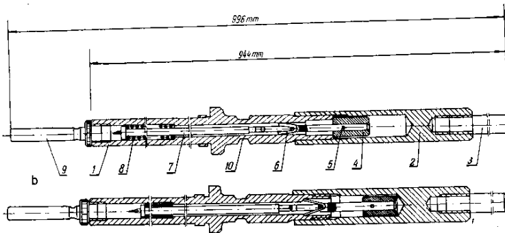
Rys. 56. MZP – przekrój.
