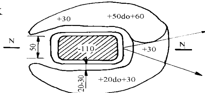
Rys. 19. Wymiary okopu strzeleckiego do strzelania: a) w postawie leżącej; b) w postawie klęczącej; c) w postawie stojącej
