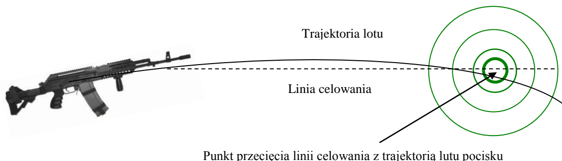
Rys .12. Odpowiednie ustawienie przyrządów celowniczych wymusza nieznaczne podniesienie broni, dzięki któremu parabola lotu pocisku przecina się z linią celowania, (która jest płaska) w punkcie wybranym przez strzelca.
