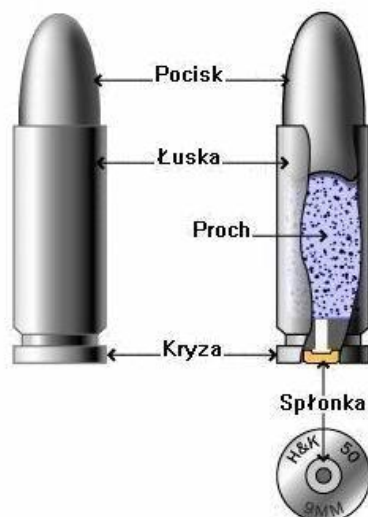
Rys. 9. Budowa naboju
